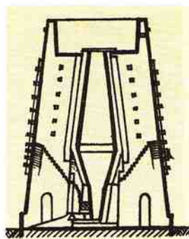
Схема устройства доменной печи
